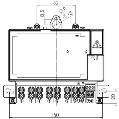
DD3 mit Zusatzklemmen
